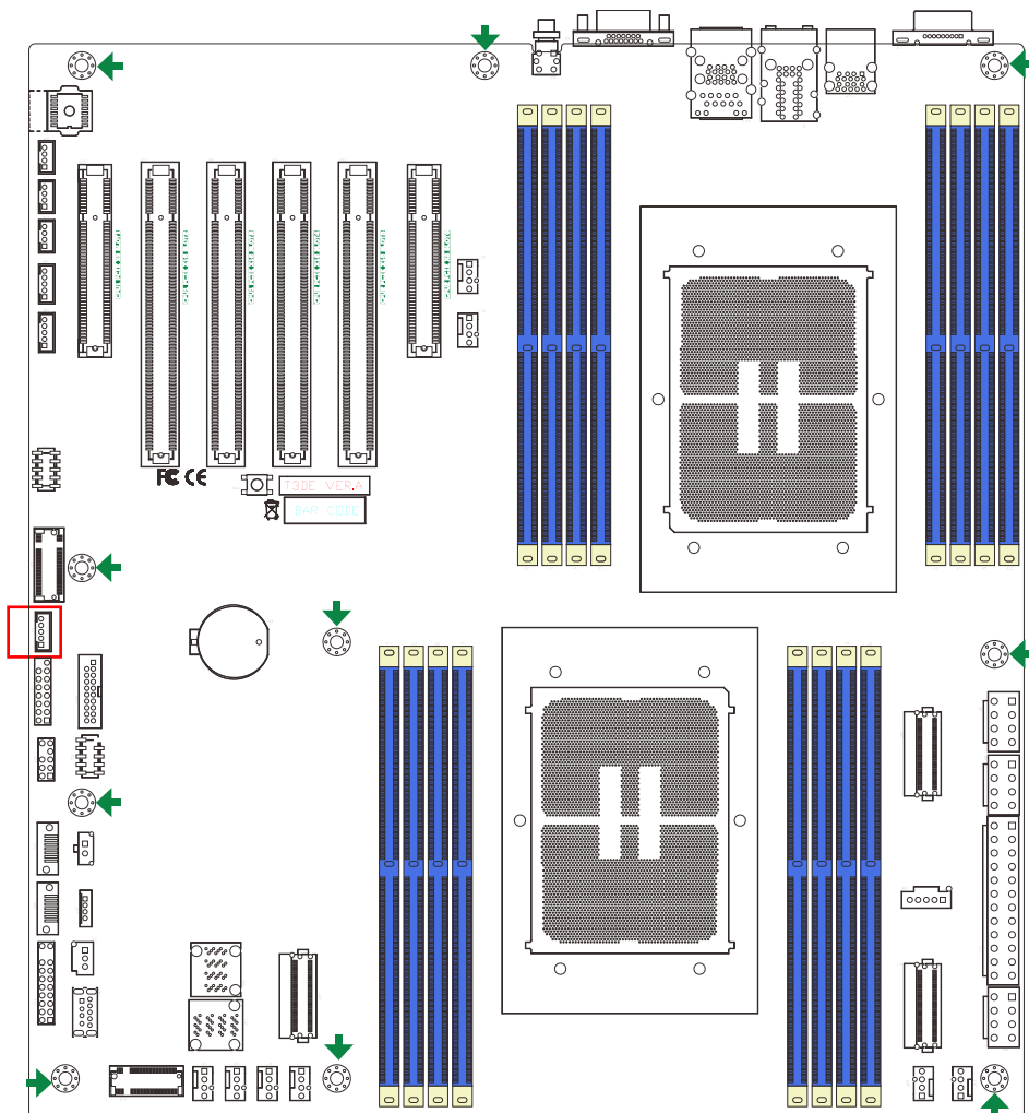
S-SGPIO Header 信号定义
