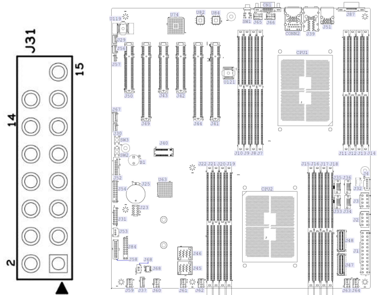
PIN 定义:
