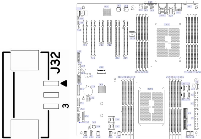
PIN 定义:
