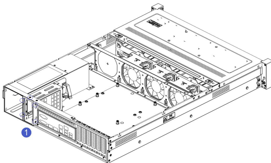
1-3.组件 2.5HDD 模块安装步骤;
